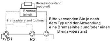
Abb. 2 für Modelle der VFD-E Serien VFD007E11A, VFD015E21A, VFD022E21A/23A/43A, VFD037E23A/43A, VFD055E23A/43A, VFD075E23A/43A, VFD110E43A
