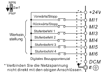
Abb. 3 Verdrahtung für den NPN-Modus und PNP-Modus
