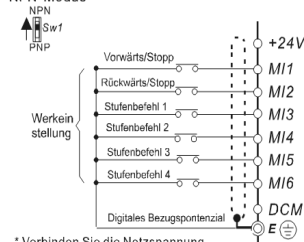
Abb. 3 Verdrahtung für den NPN-Modus und PNP-Modus
